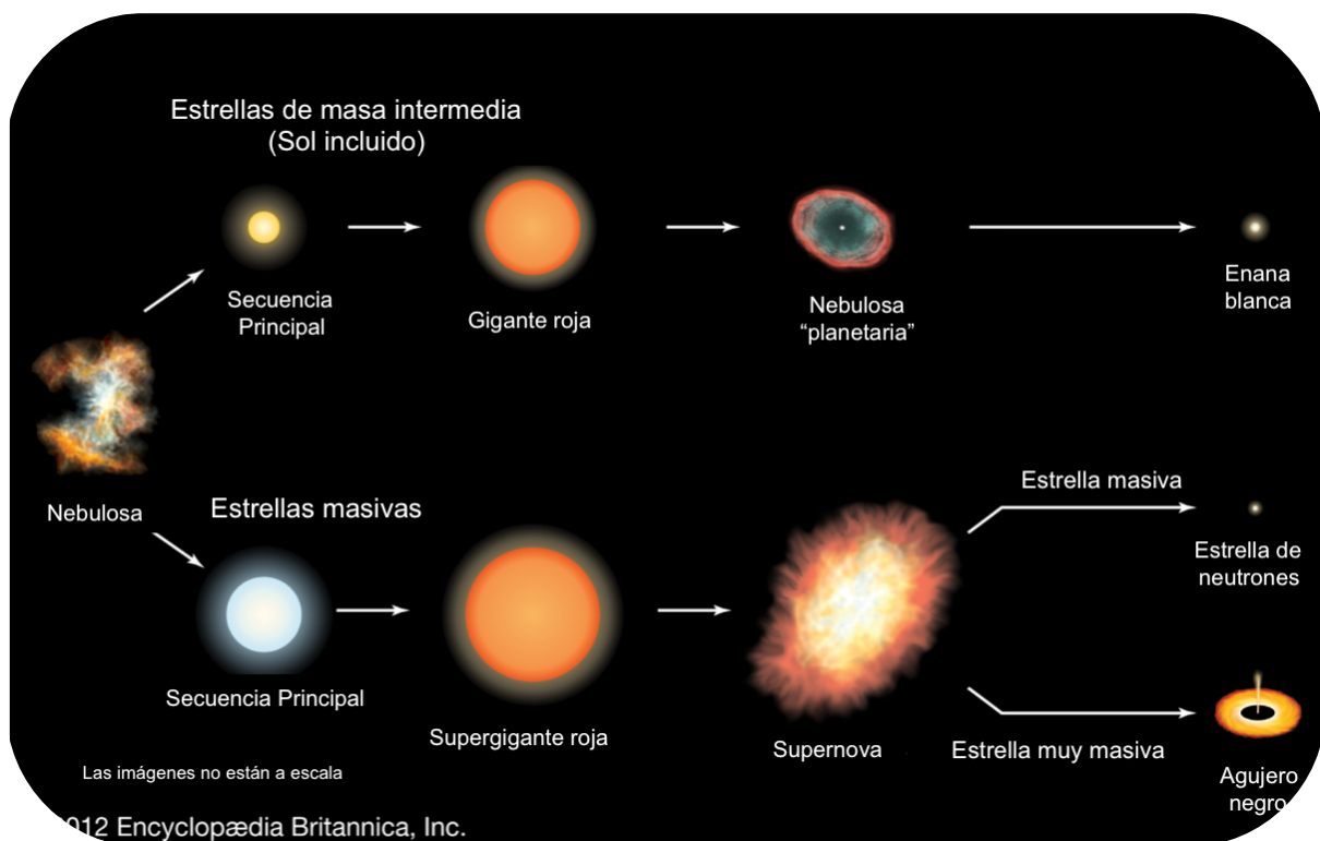
Figura 5: La evolución de una estrella depende de su masa. (Crédito: Encyclopædia Britannica)
