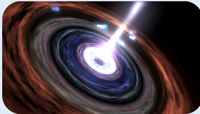
Un núcleo activo de galaxia o AGN (Crédito: NASA)
