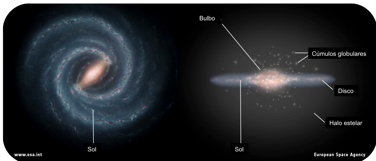
Figura 2: Estructura de una galaxia espiral, la Vía Láctea. (Crédito: ESA)
