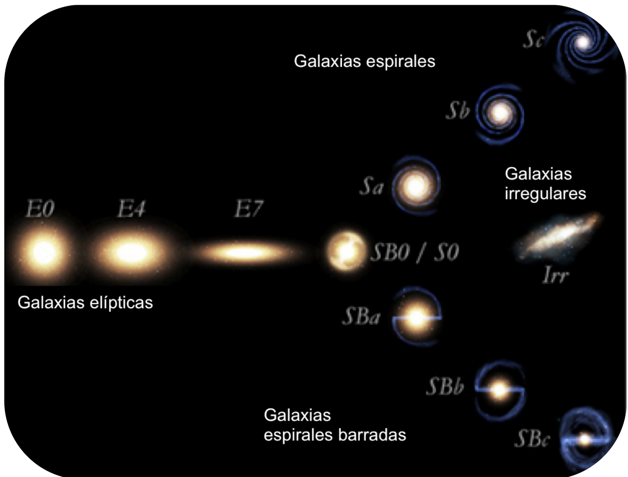
Figura 1: Diagrama de horca de Hubble. (Crédito: NASA/ESA)
